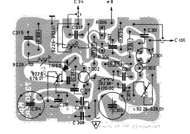
Mischteil, Bestückungsseite MIXER STAGE PRINTED BOARD, COMPONENT SIDE MELANGEUR, VUE DU COTE DES COMPOSANTS PARTE MISCELATRICE, LATO COMPONENTI
